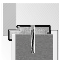
rohová zárubeň velká montáž pomocí šroubů
